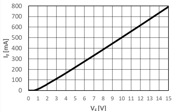
図2. ブートストラップDi V_F - I_F 代表特性(制限抵抗による電圧降下含む)(右図は拡大図)
