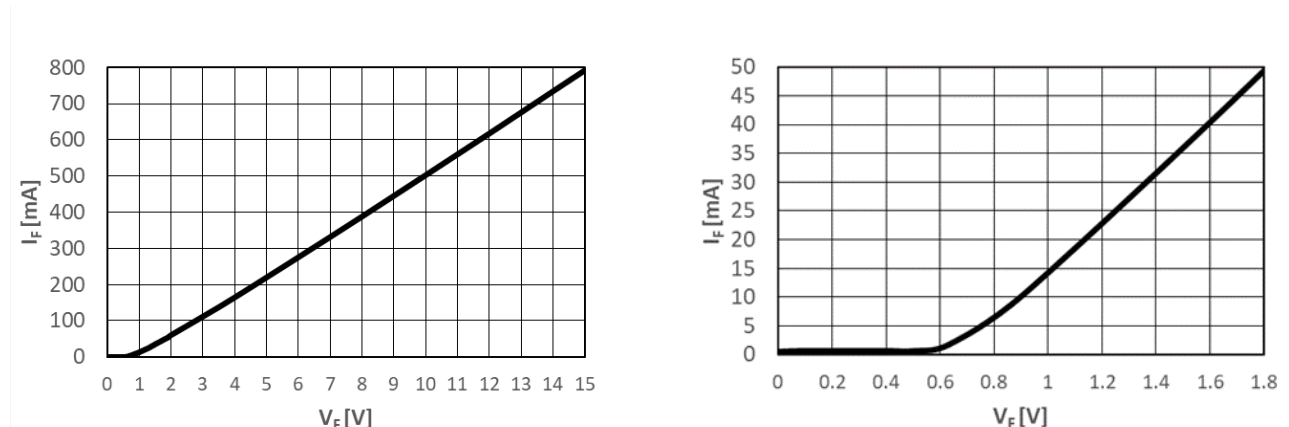
図2. ブートストラップDi V_F - I_F 代表特性(制限抵抗による電圧降下含む)(右図は拡大図)
