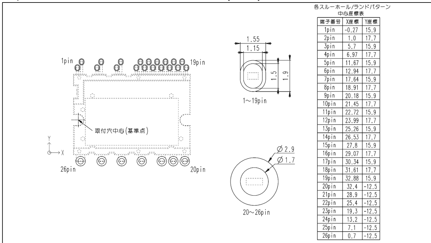
図11. (参考図)PCBレイアウトパターン
