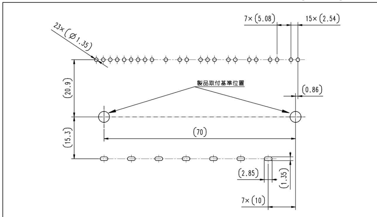
図9. (参考図) PCB スルーホールパターン
