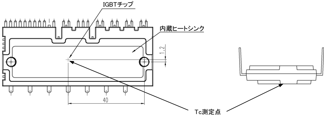
図1. ケース温度 T_C 測定点
