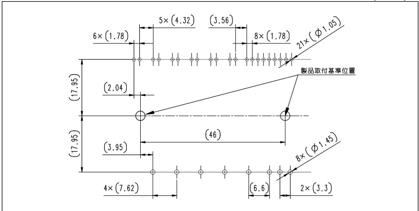
図10. (参考図) PCB スルーホールパターン
