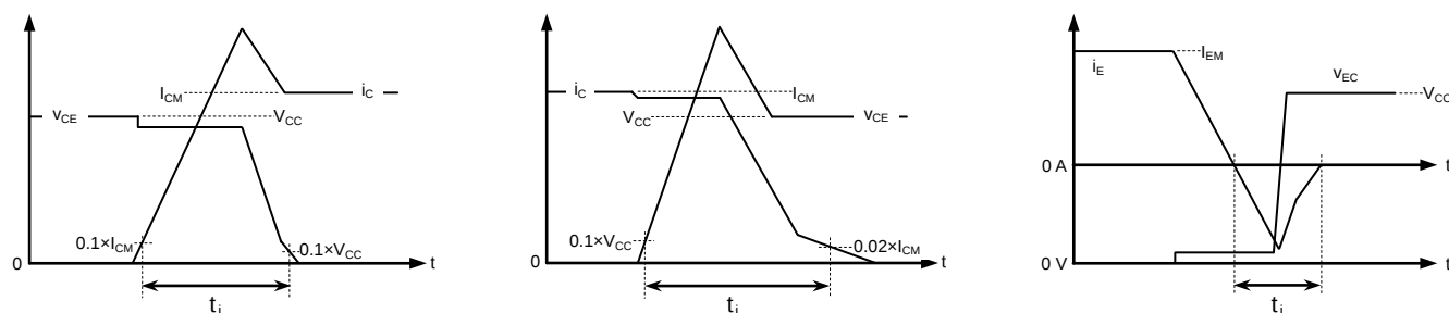
IGBT ターンオンスイッチング損失
