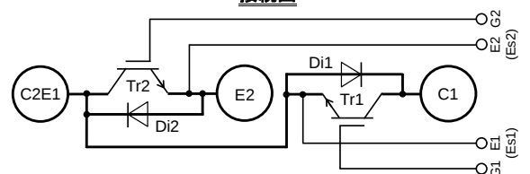
接続図
