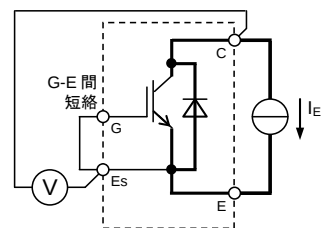
V_{EC} 試験回路
