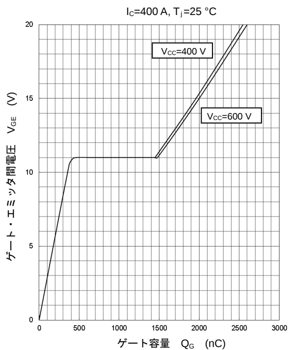
ゲート容量特性 (代表例)
