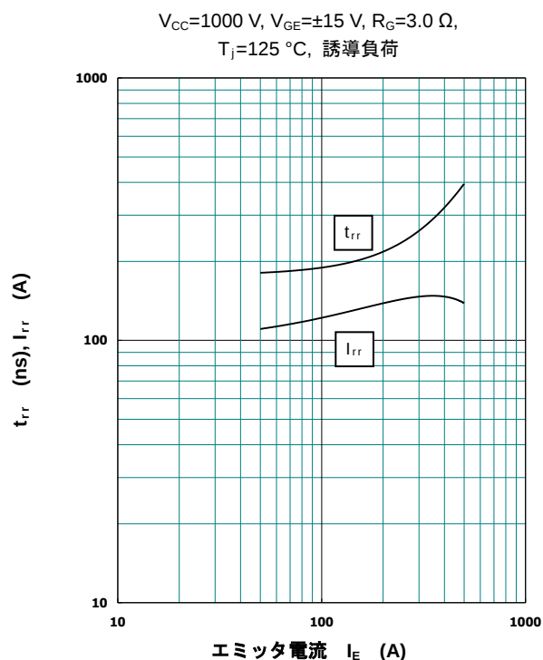
フリーホイールダイオード逆回復特性 (代表例)
