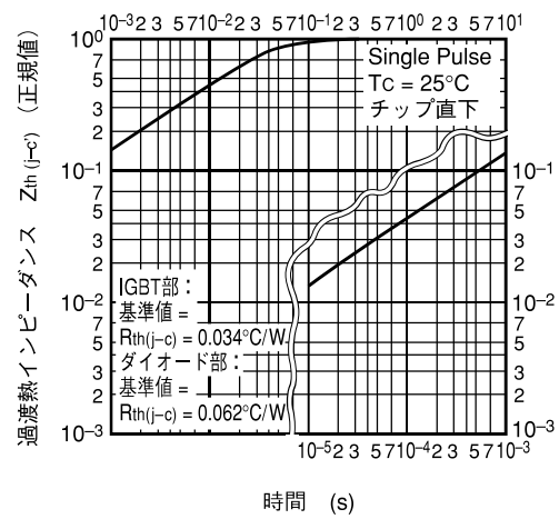
過渡熱抵抗特性 (IGBT部, ダイオード部)
