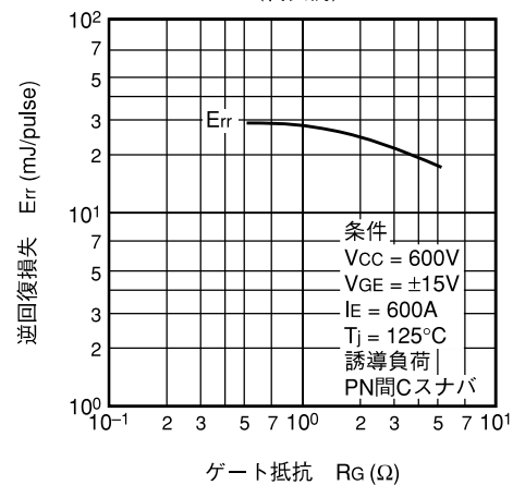
逆回復損失特性 ( Err-R_G ) (代表例)
