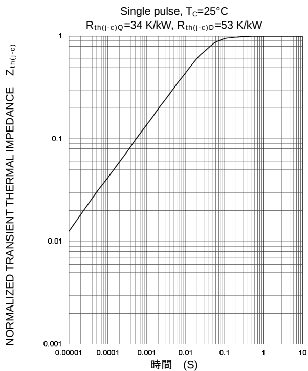
最大過渡熱インピーダンス特性 (最大値)
