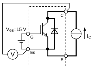
V_{CEsat} 試験回路
