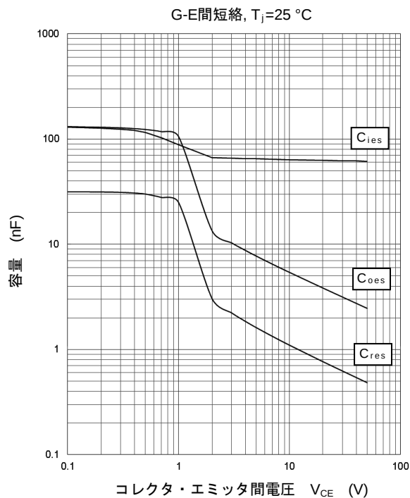
ゲート容量特性 (代表例)
