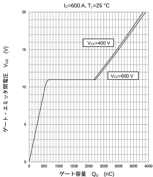
ゲート容量特性 (代表例)
