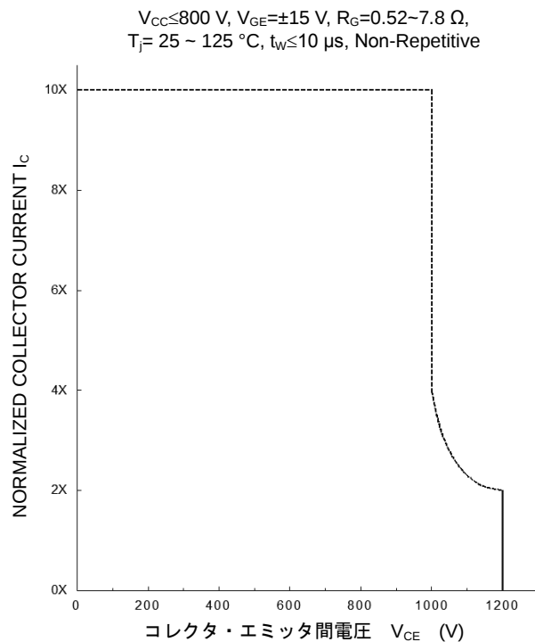
短絡安全動作領域 (最大値)
