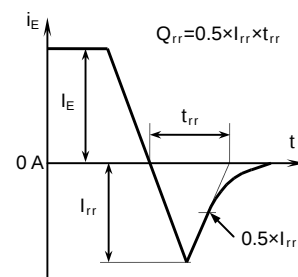
逆回復特性試験波形
