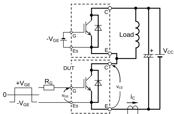
スイッチング特性試験回路及び試験波形
