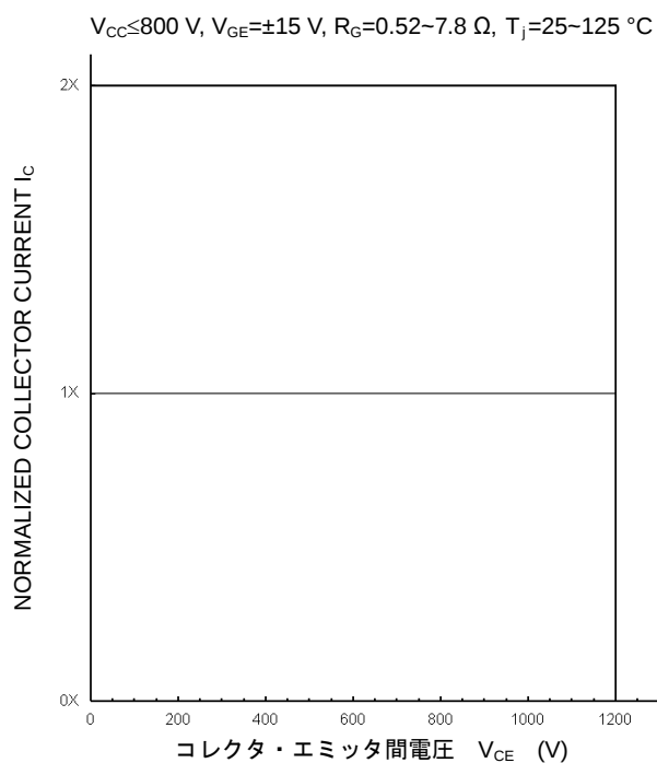
ターンオフスイッチング安全動作領域 (逆バイアス安全動作領域) (最大値)
