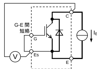
V_{EC} 試験回路
