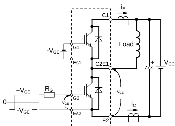
スイッチング特性試験回路及び試験波形
