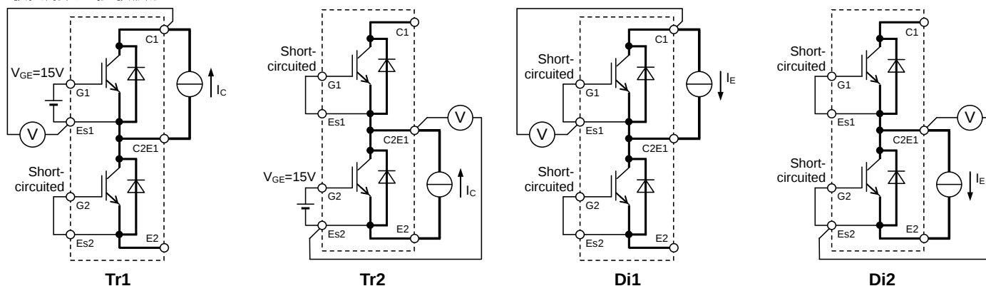
V_{CEsat} 試験回路
