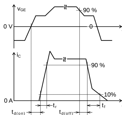
スイッチング特性試験回路及び試験波形
