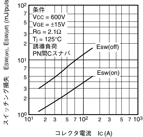
スイッチング損失特性 ( E_{sw(on)} , E_{sw(off)} - I_C ) (代表例)
