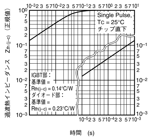
過渡熱抵抗特性 (IGBT部, ダイオード部)
