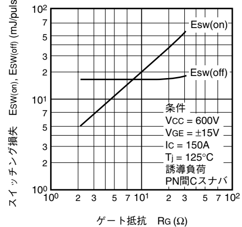
スイッチング損失特性 ( E_{sw(on)} , E_{sw(off)} - R_G ) (代表例)
