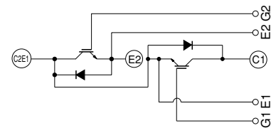
接続図 CIRCUIT DIAGRAM
