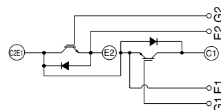
接続図 CIRCUI T DIAGRAM
