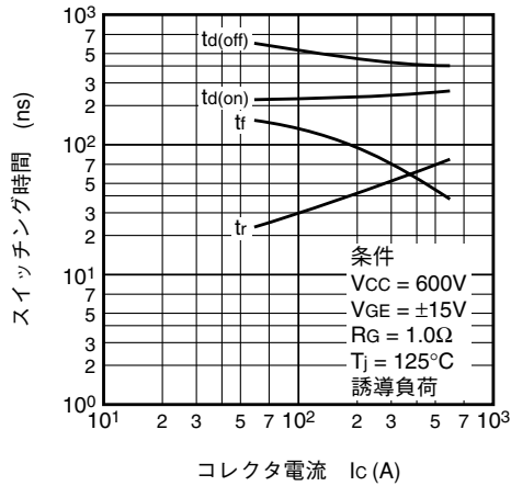
ハーフブリッジスイッチング特性 (代表例)
