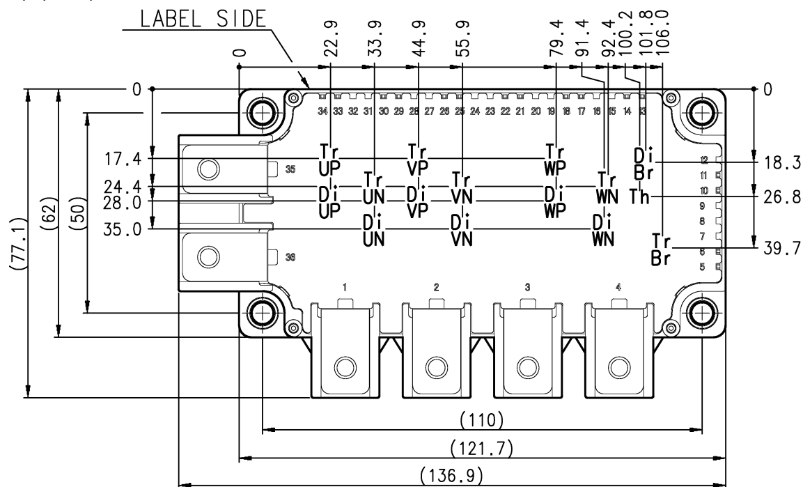
チップ配置図 (Top view)
