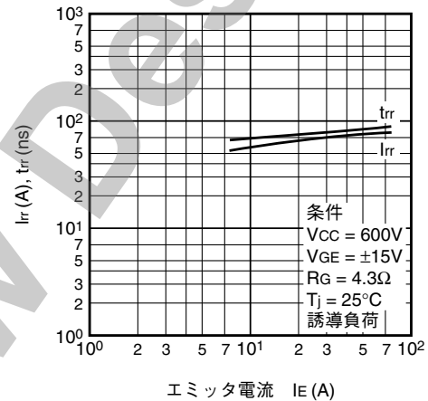
ダイオード部回復特性 (代表例) インバータ部
