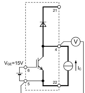
ブレーキ IGBT
