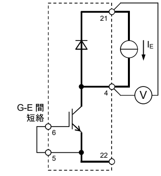
ブレーキ DIODE
