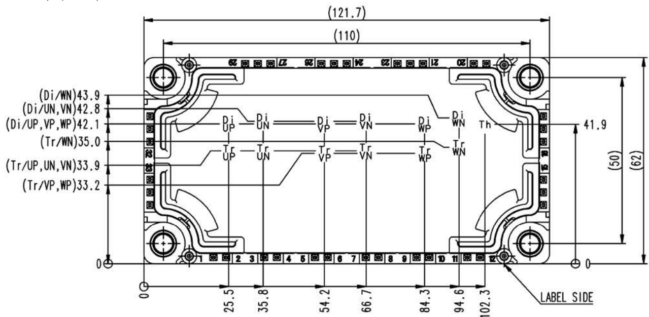
チップ配置図 (Top view)
