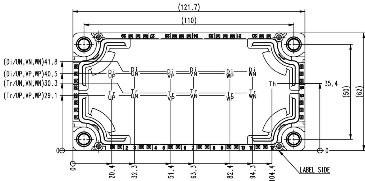
チップ配置図 (Top view)
