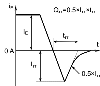
逆回復特性試験波形
