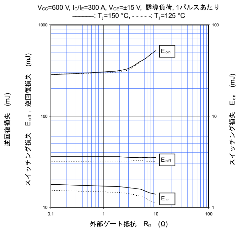
スイッチング損失特性 (代表例)
