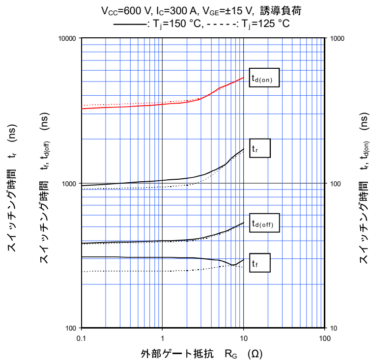
スイッチング時間特性 (代表例)
