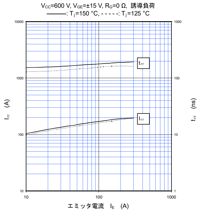
フリーホイールダイオード逆回復特性 (代表例)
