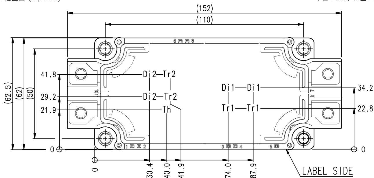
單位：mm，公差：±1 mm
