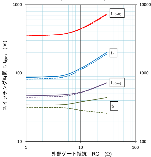
スイッチング時間特性 (代表例)
