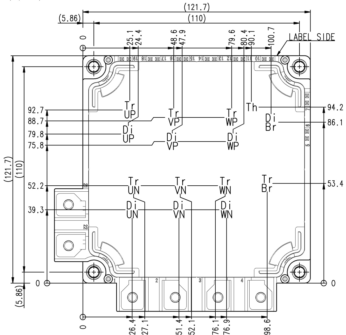
チップ配置図 (Top view)
