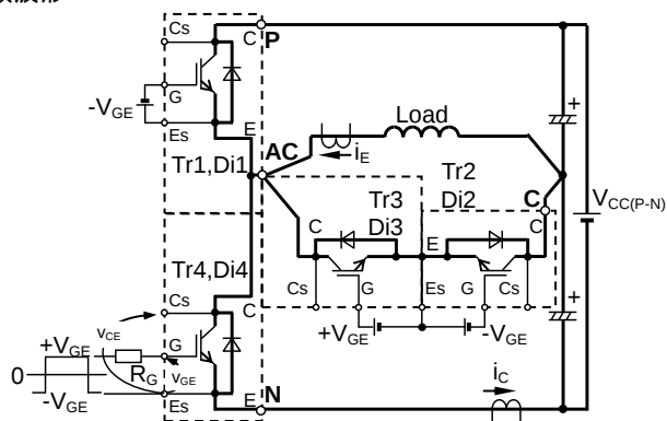
スイッチング特性試験回路及び試験波形 (BRIDGE 部スイッチング)
