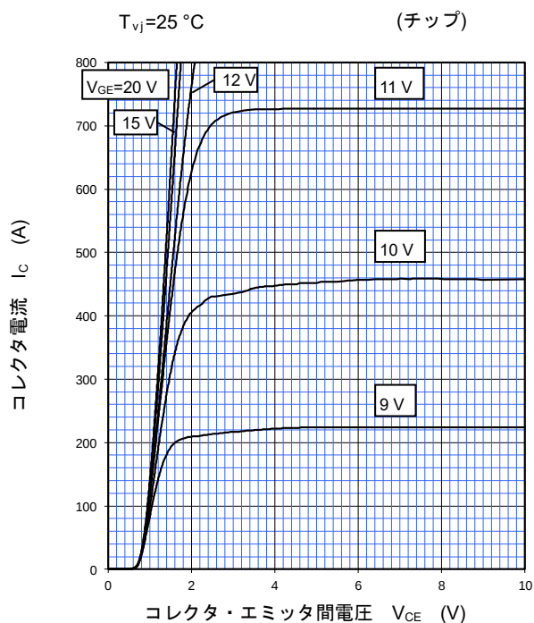
コレクタ・エミッタ間飽和電圧 (代表例)
