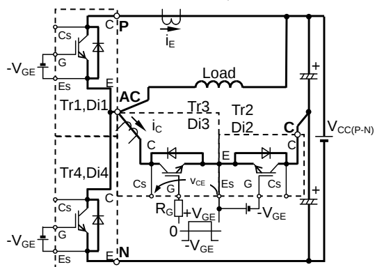
スイッチング特性試験回路及び試験波形 (AC SWITCH 部スイッチング)
