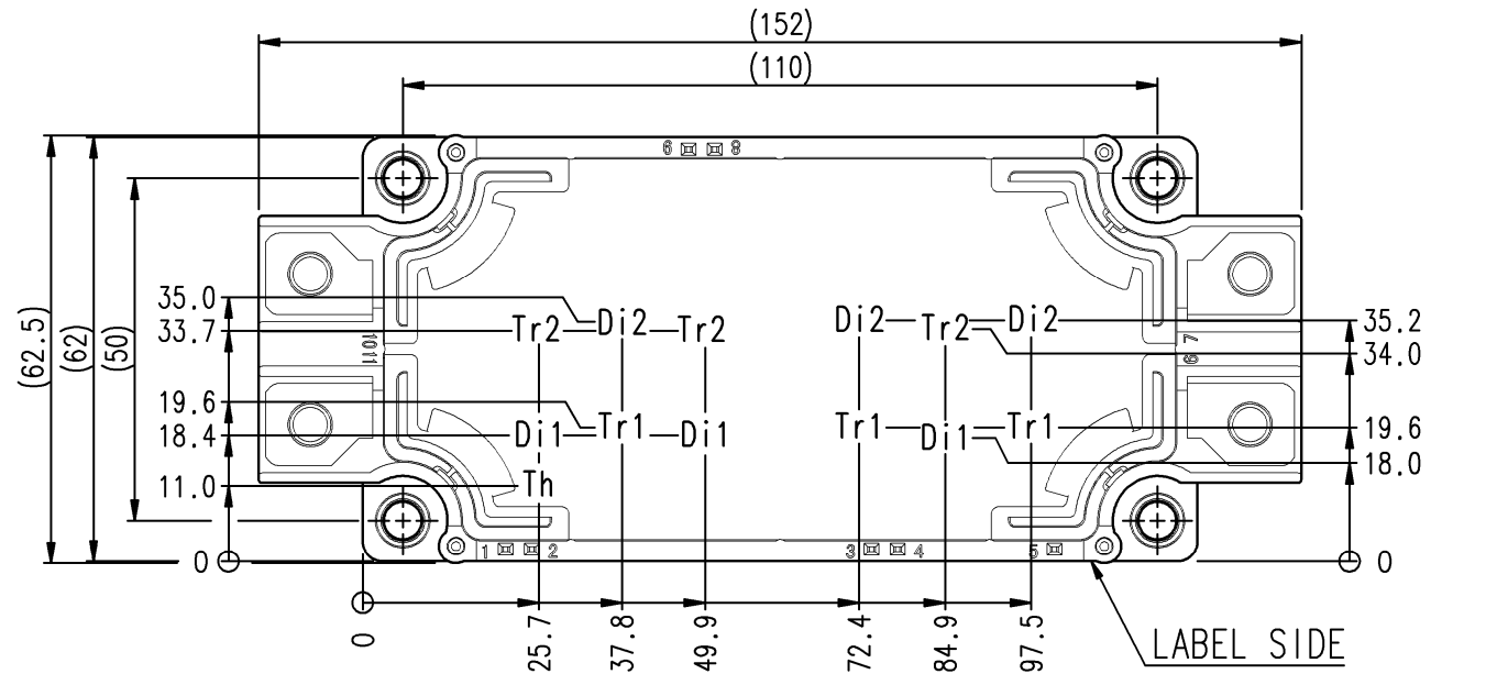
チップ配置図 (Top view)
