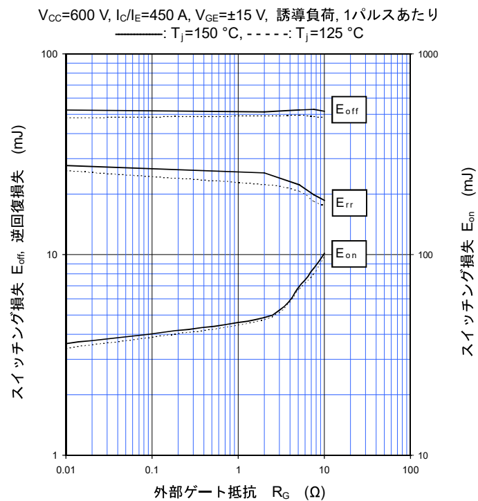
スイッチング損失特性 (代表例)
