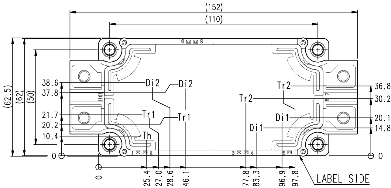
チップ配置図 (Top view)
