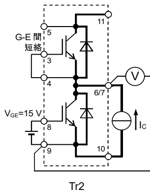
V_{CEsat} 試験回路
