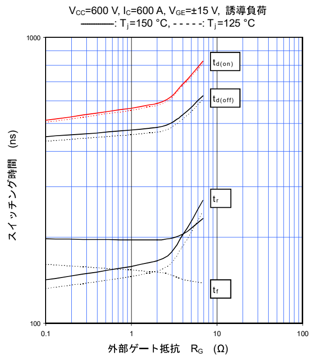
スイッチング時間特性 (代表例)
