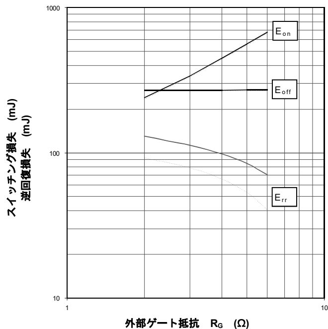
スイッチング損失特性 (代表例)
