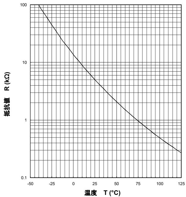
温度特性 (代表例)
