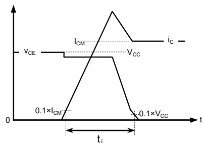
IGBT ターンオンスイッチング損失
