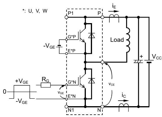
スイッチング特性試験回路及び試験波形
