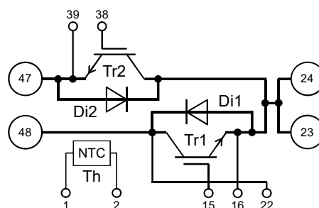
接続図
