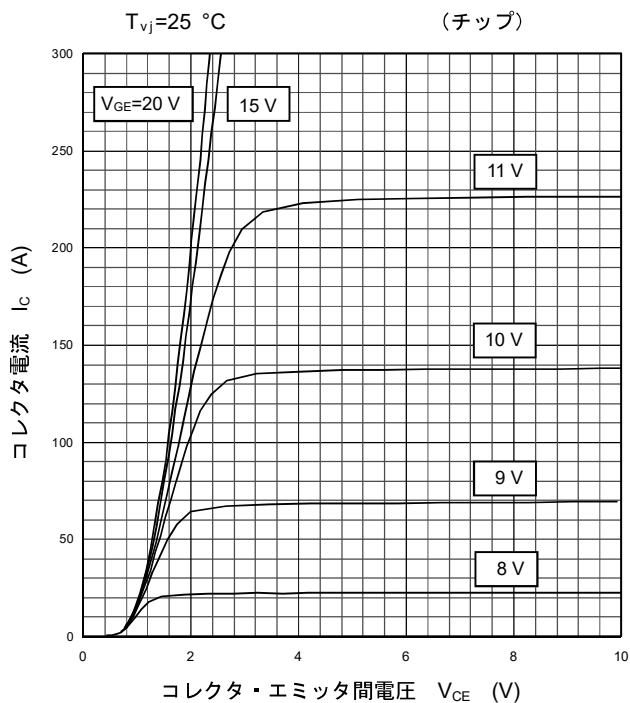
出力特性 (代表例)
