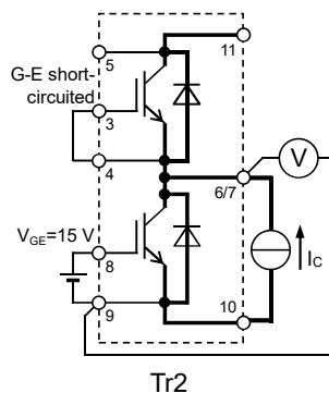
V_{CEsat} 試験回路
