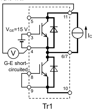
V_{CEsat} 試験回路
