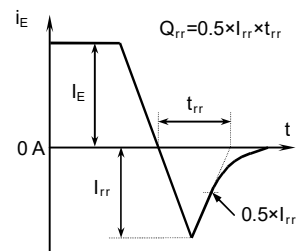
逆回復特性試験波形
