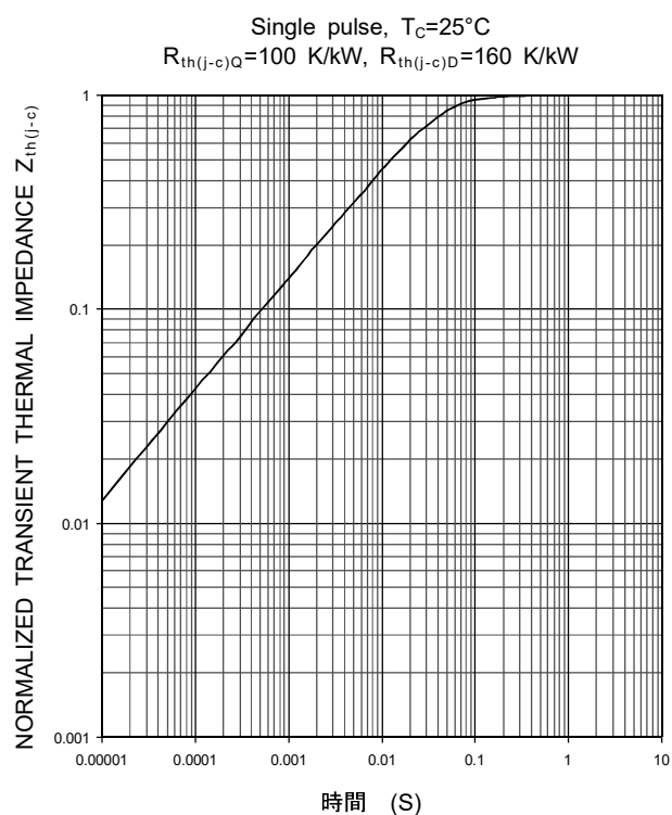
過渡熱インピーダンス特性 (最大)
