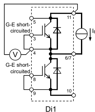
V_{EC} 試験回路
