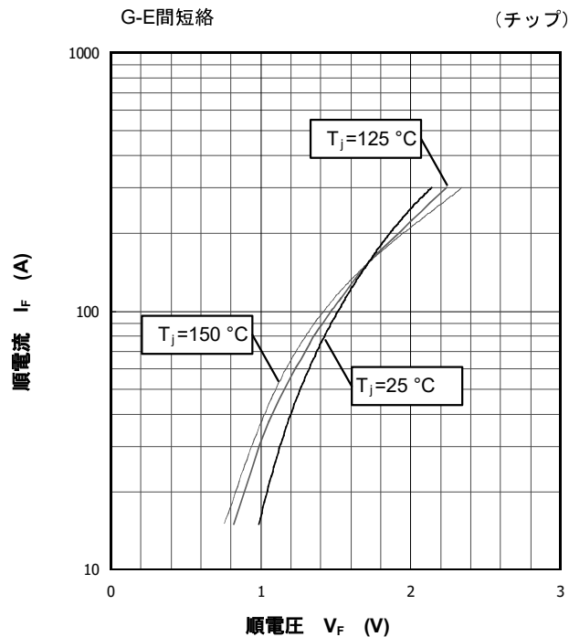
ダイオード順特性 (代表例)
