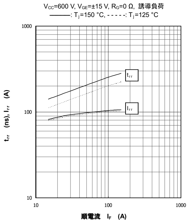
ダイオード逆回復特性 (代表例)
