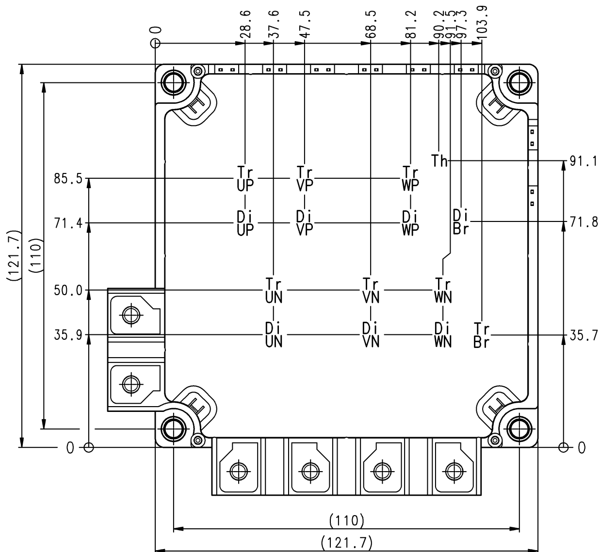
チップ配置図 (Top view)
