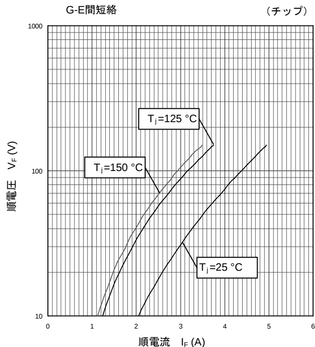
スイッチング損失特性 (代表例)
