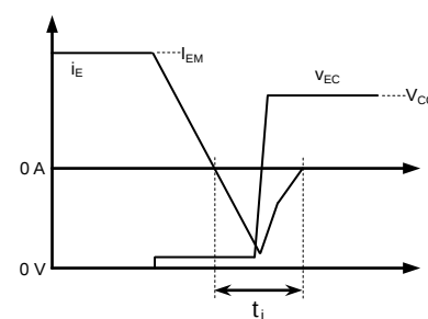
FWD 逆回復損失
