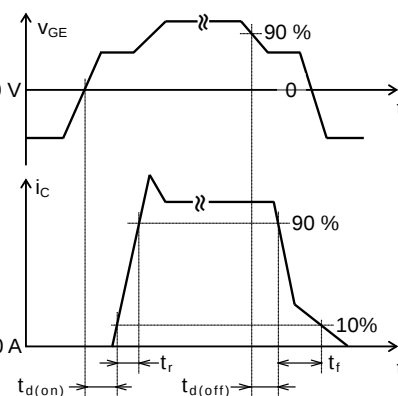
スイッチング特性試験回路及び試験波形
