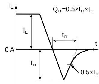
逆回復特性試験波形
