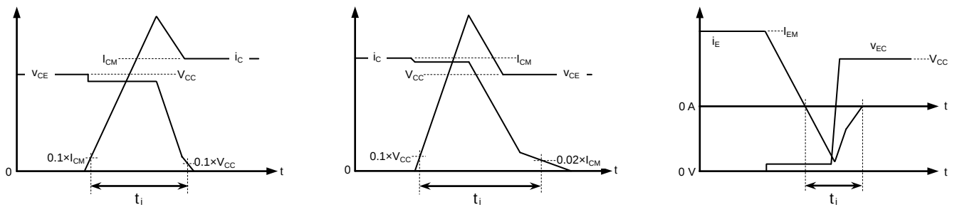
ターンオン / ターンオフスイッチング損失及び逆回復損失試験波形（積分時間説明図）
