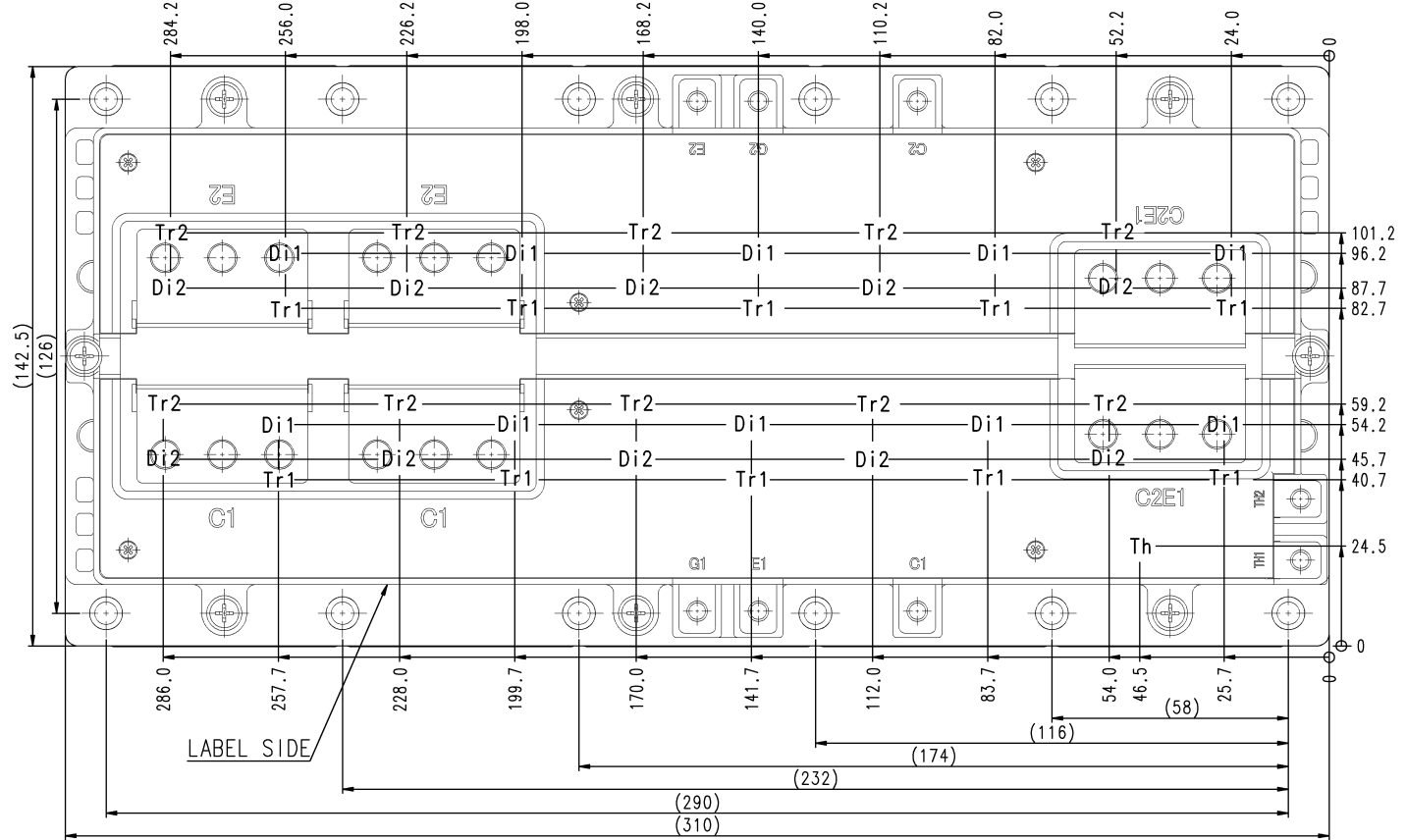
チップ配置図 (Top view)
