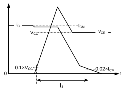
スイッチング損失及び逆回復損失試験波形（積分時間説明図）
