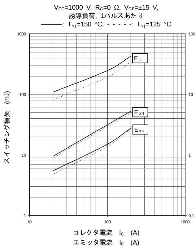
スイッチング損失特性 (代表例)
