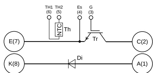
接続図
