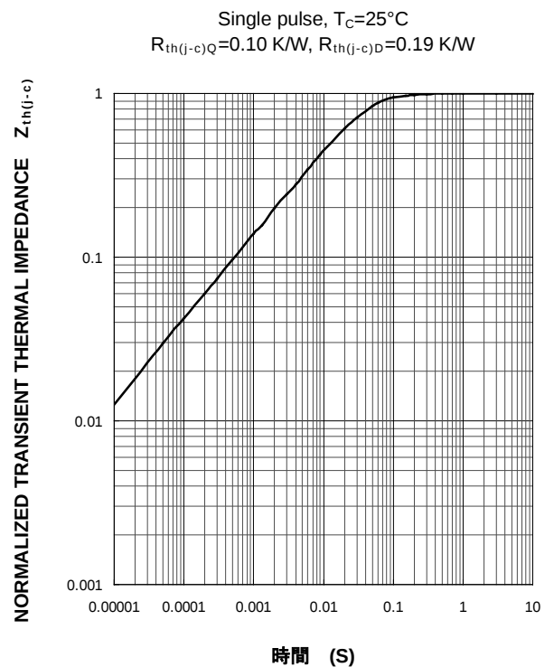
最大過渡熱インピーダンス特性
