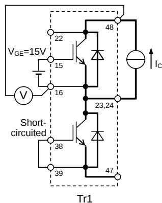
V_{CEsat} 試験回路
