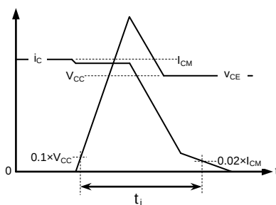
IGBT ターンオフスイッチング損失
