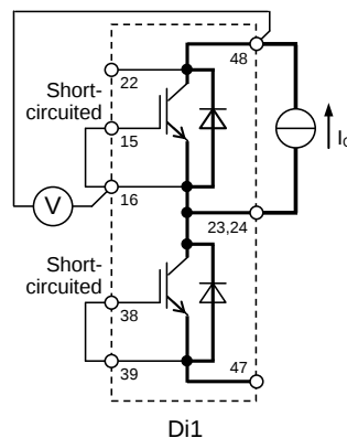
V_{EC} 試験回路
