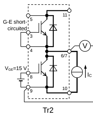
V_{CEsat} 試験回路
