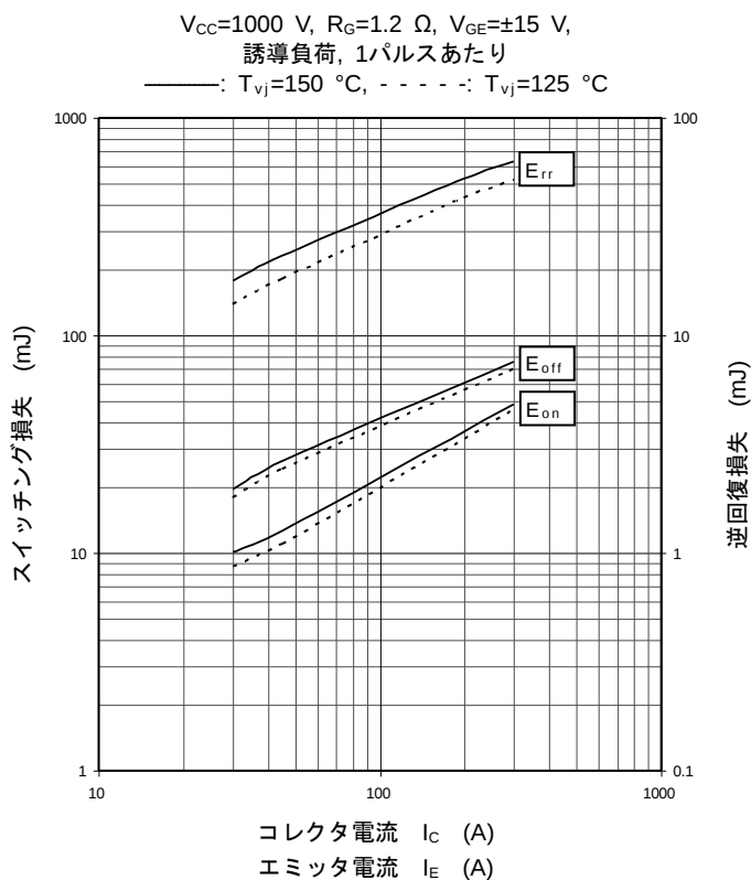
スイッチング損失特性 (代表例)
