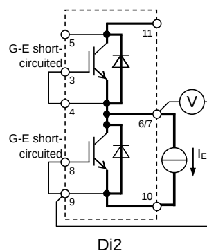
V_{EC} 試験回路
