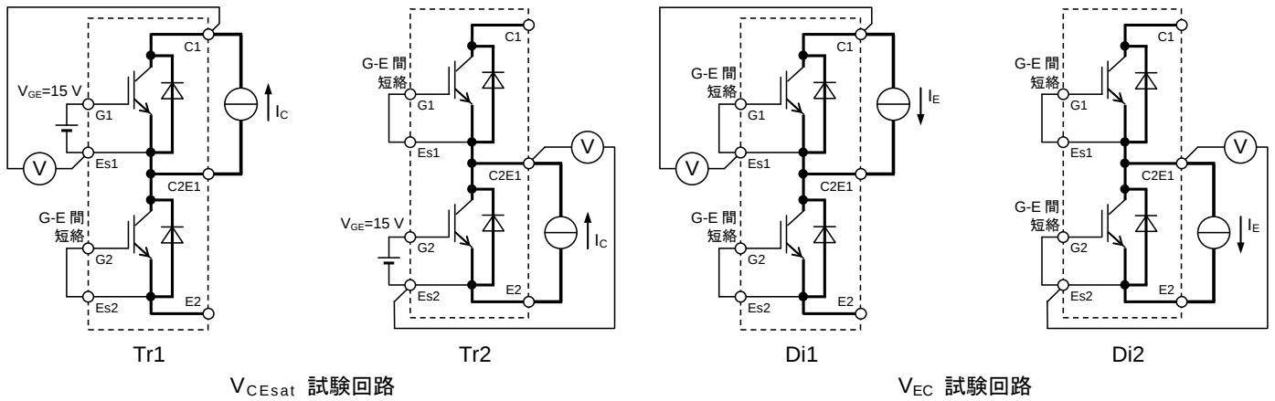
試験回路
