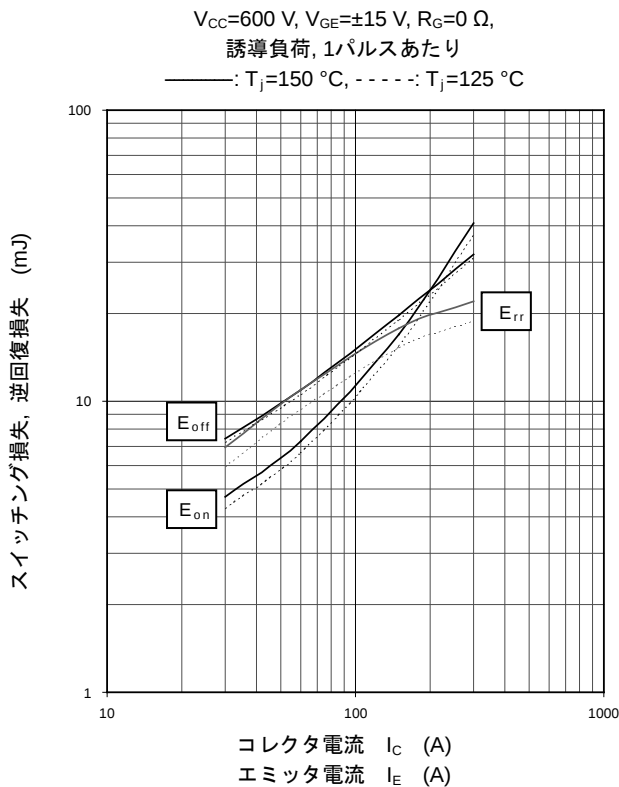
スイッチング損失特性 (代表例)
