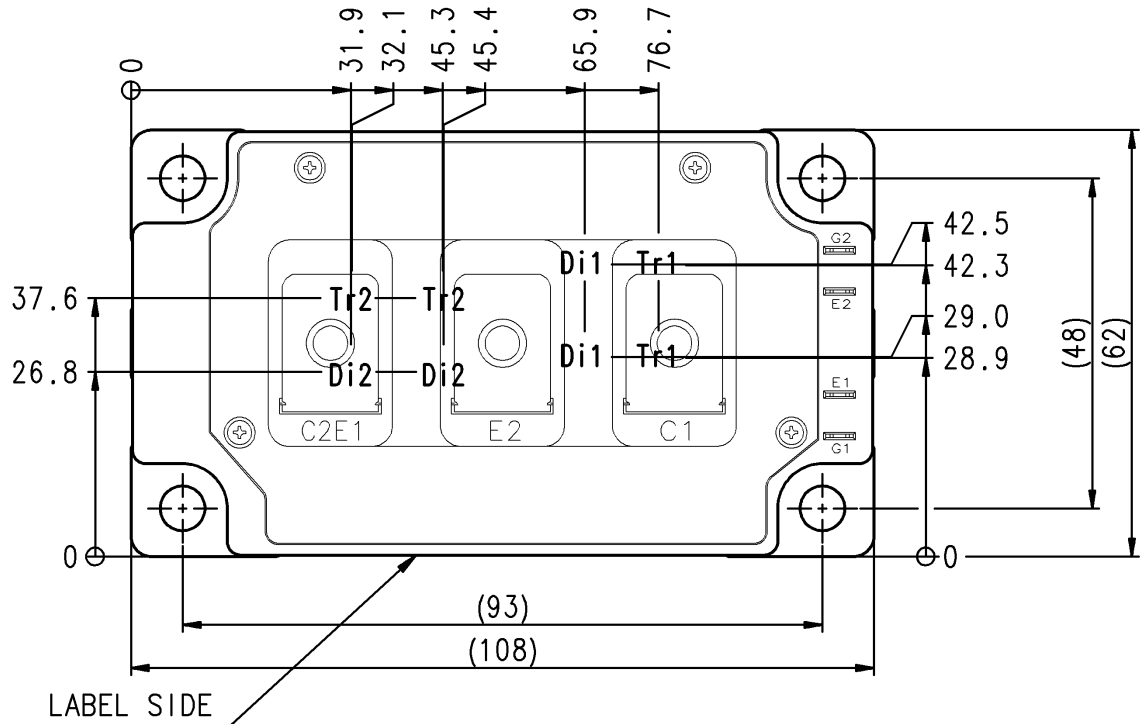
チップ配置図 (Top view)
