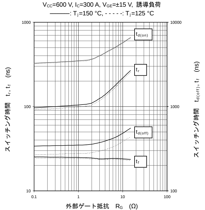
スイッチング時間特性 (代表例)
