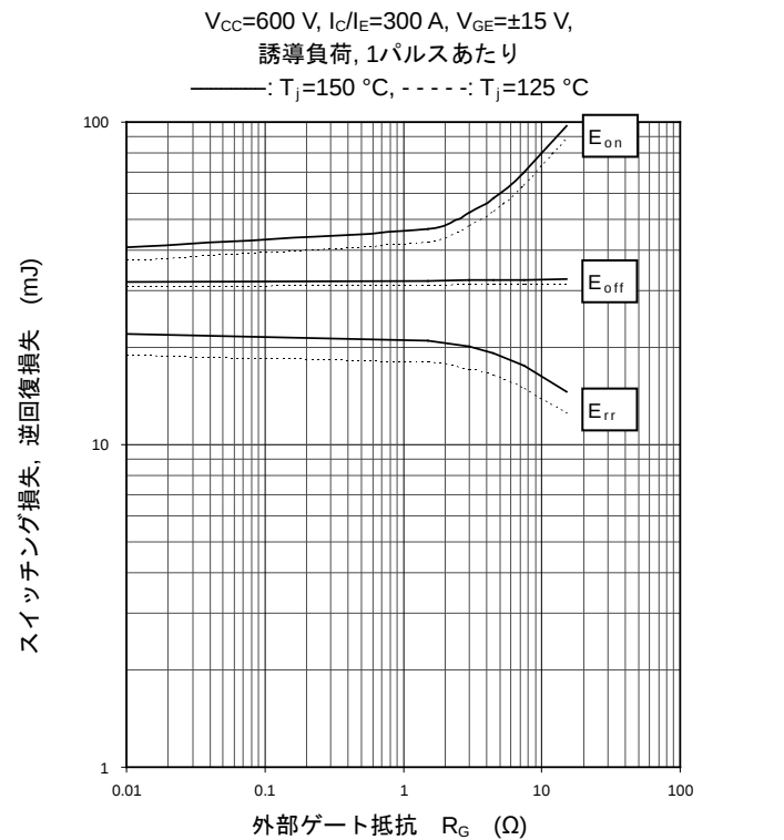
スイッチング損失特性 (代表例)
