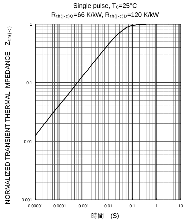
最大過渡熱インピーダンス特性
