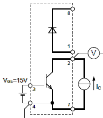
V_{CEsat} 試験回路
