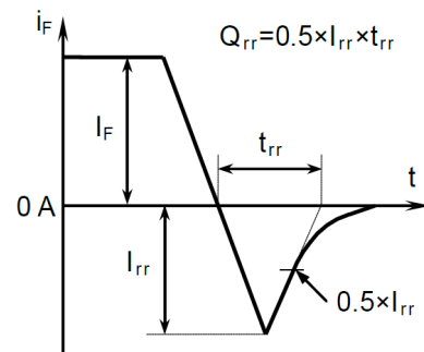
逆回復特性試験波形
