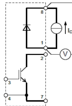
V_F 試験回路
