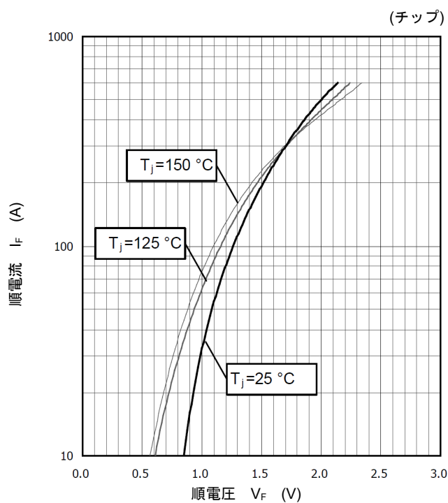
ダイオード順特性 (代表例)
