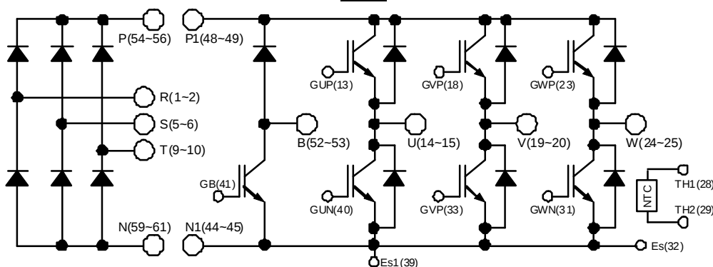
接続図
