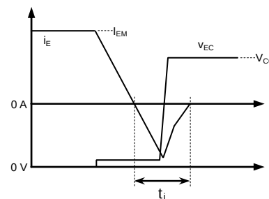
FWD 逆回復損失
