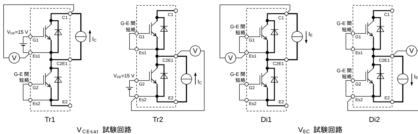
試験回路
