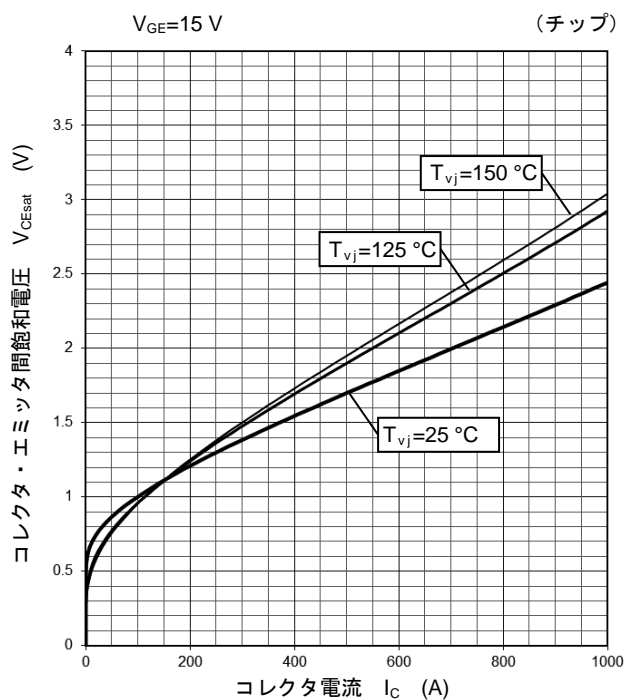
コレクタ・エミッタ飽和電圧特性 (代表例)
