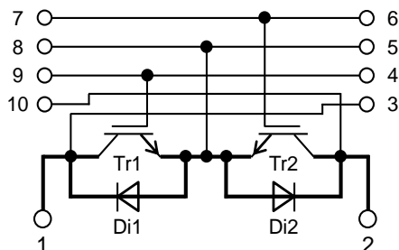
内部接続図
