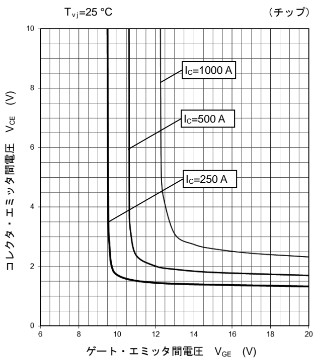
コレクタ・エミッタ間電圧特性 (代表例)
