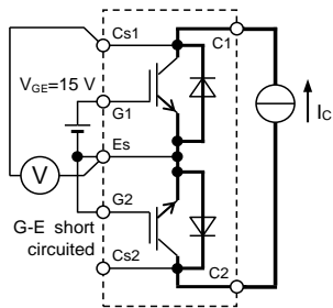
V_{CEsat} 試験回路
