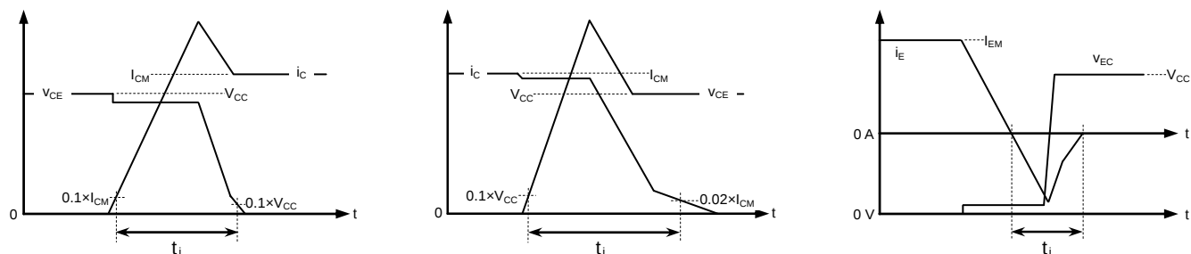
IGBT ターンオンスイッチング損失
