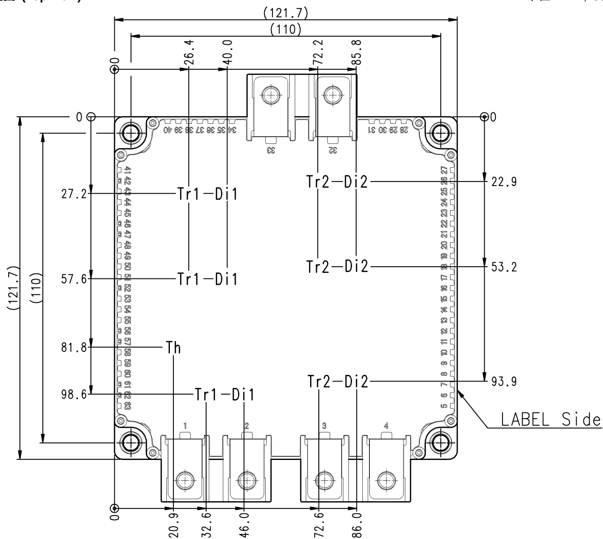
チップ配置図 (Top view)
