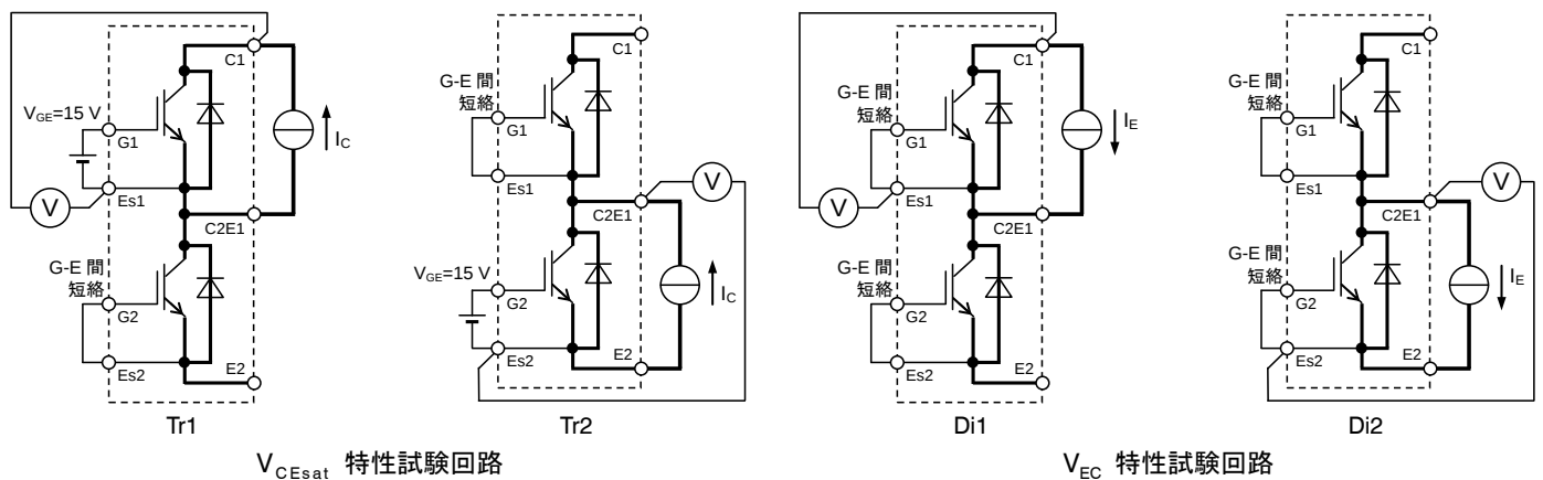
試験回路
