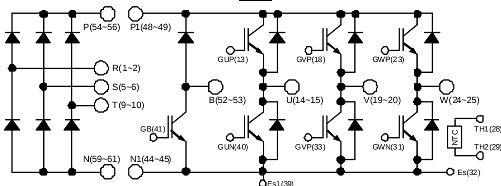
接続図
